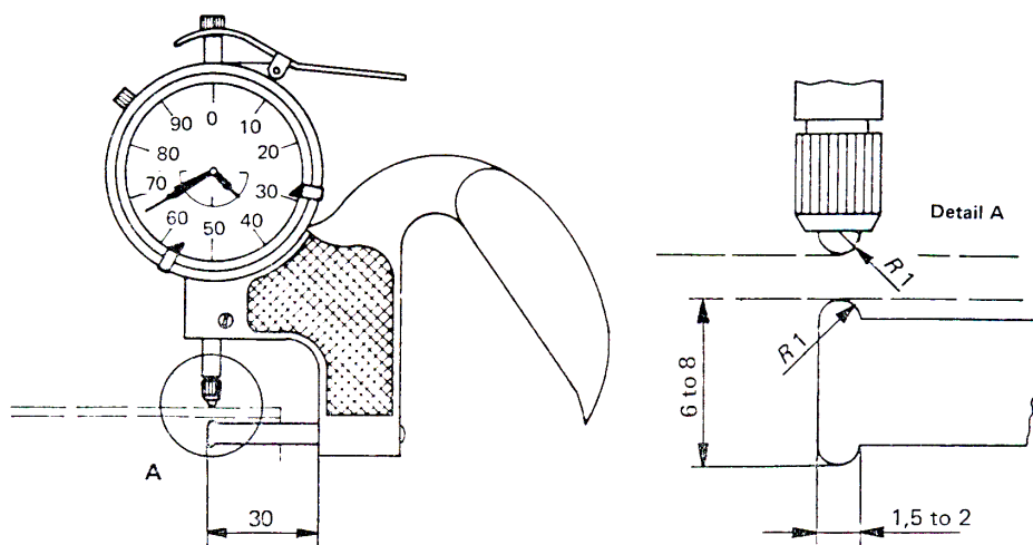
شکل ۱- وسیله برای اندازه گیری ضخامت لوله ها
