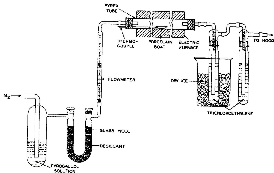
شکل یک- دستگاه اندازه گیری نیتروژن
